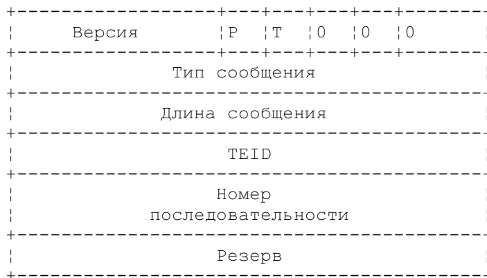
Рисунок 1. Общий формат заголовка сообщений протокола GTPv2-C
