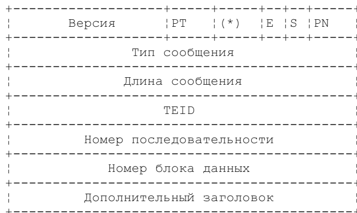
Рисунок 2. Общий формат заголовка сообщений протокола GTPv1-U
